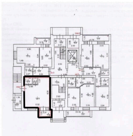
План части нежилого помещения -1, расположенного по адресу: РМЭ, г. Йошкар-Ола, ул. Аппикова, д.19
